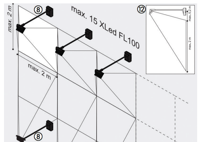
Placering och utsättning av XLED FL 100
