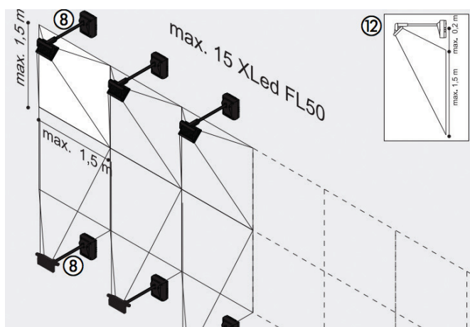
Placering och utsättning av XLED FL 50
